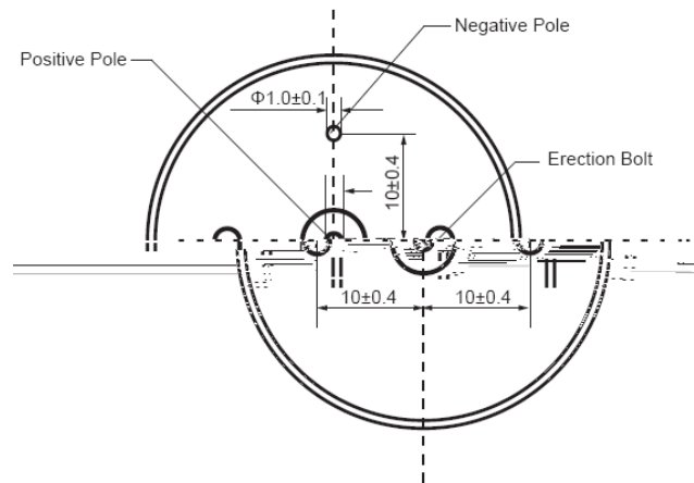
THC3W \Phi 36x20/24outline Unit:mm
